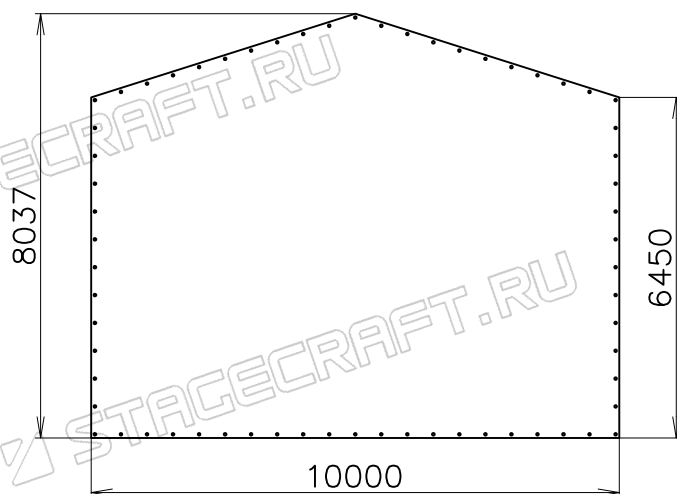
Выкройка заднего баннера
