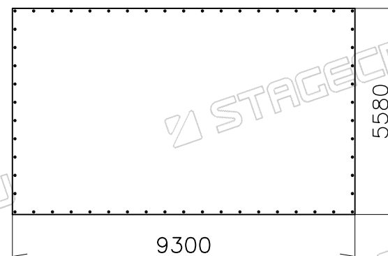
Выкройка заднего баннера
