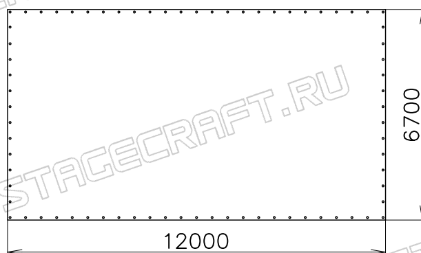
Выкройки фронтон задний баннер
