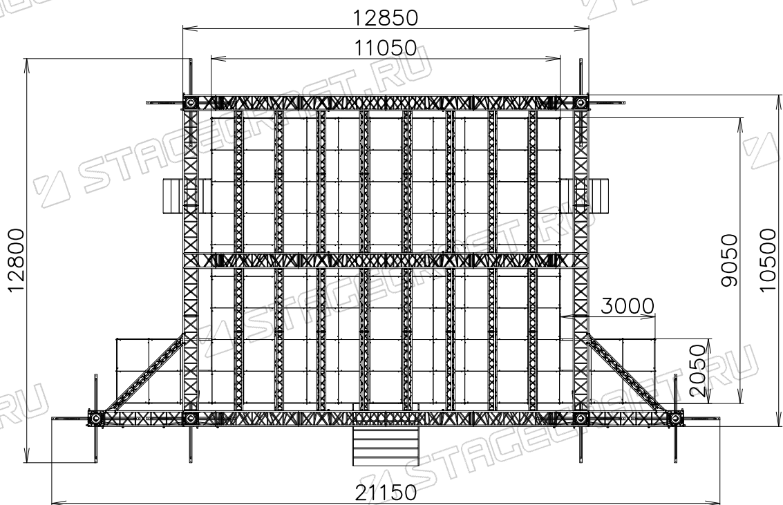
Выкройки фронтон задний баннер
