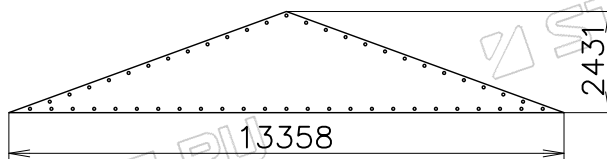
Выкройки фронтон
