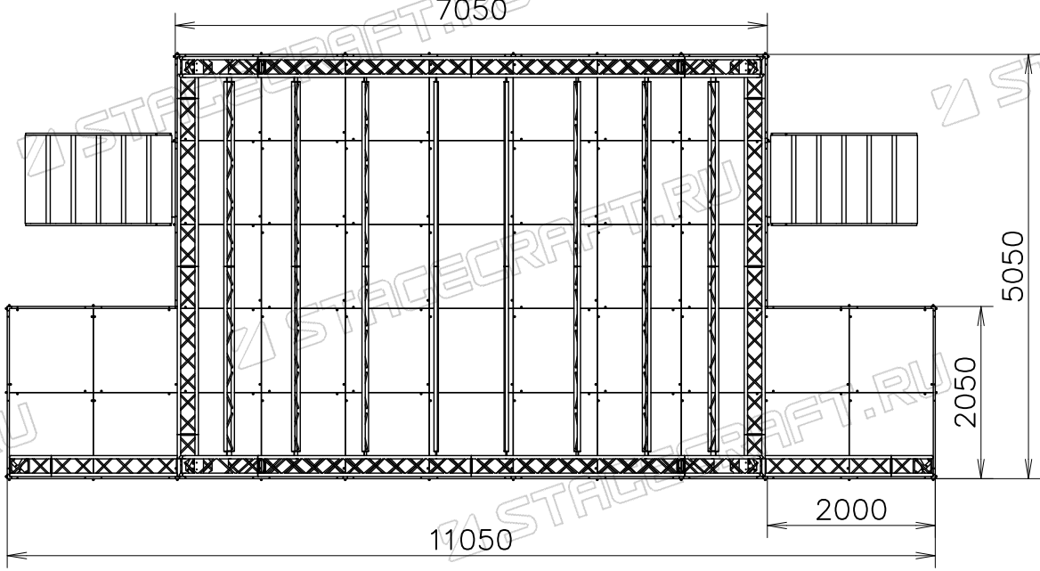
Выкройки фронтон
