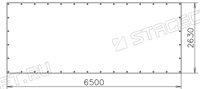
Выкройка заднего баннера
