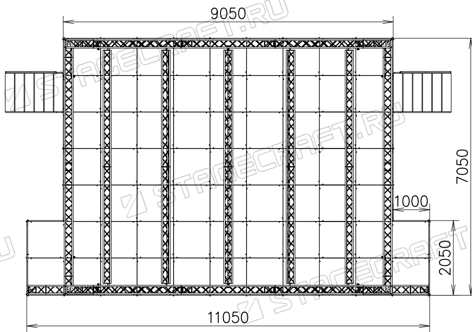
Выкройки фронтон
